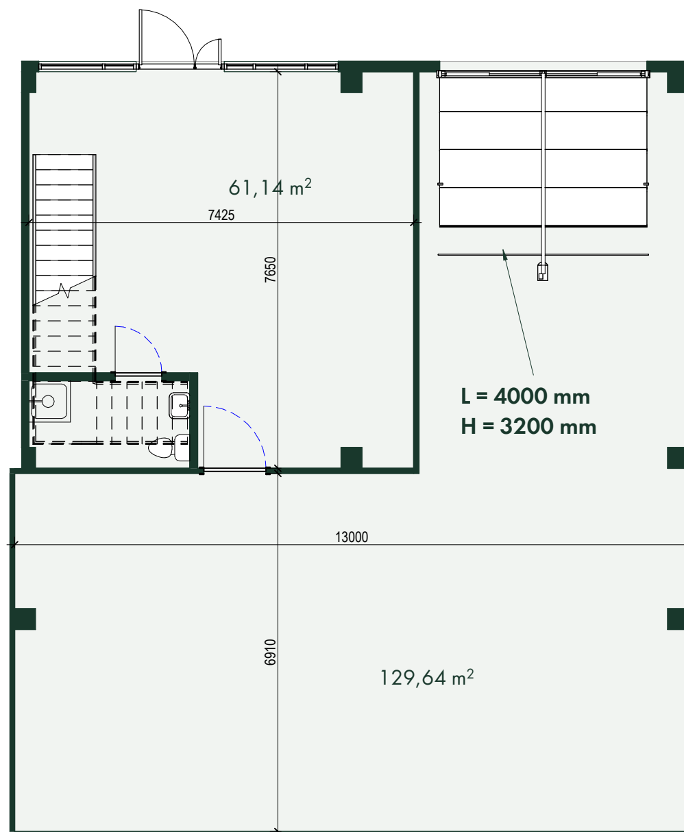
1. STĀVA PLĀNS 1. FLOOR PLAN
