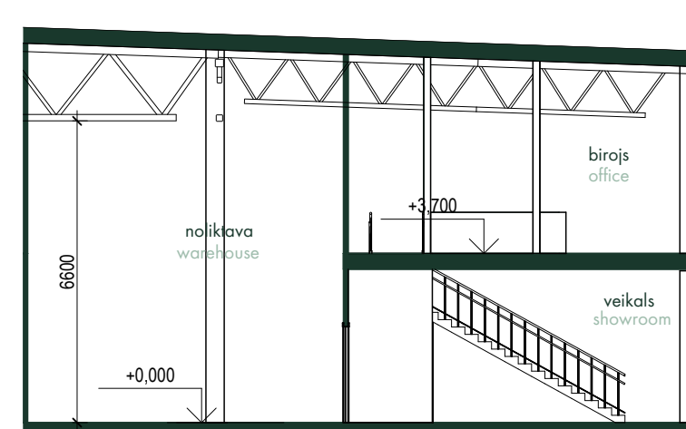
ŠĶĒRSGRIEZUMS 1-1 SECTION 1-1
