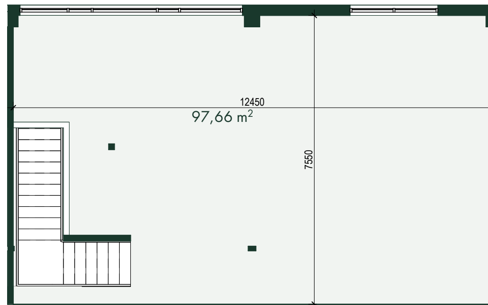
2. STĀVA PLĀNS 2. FLOOR PLAN
