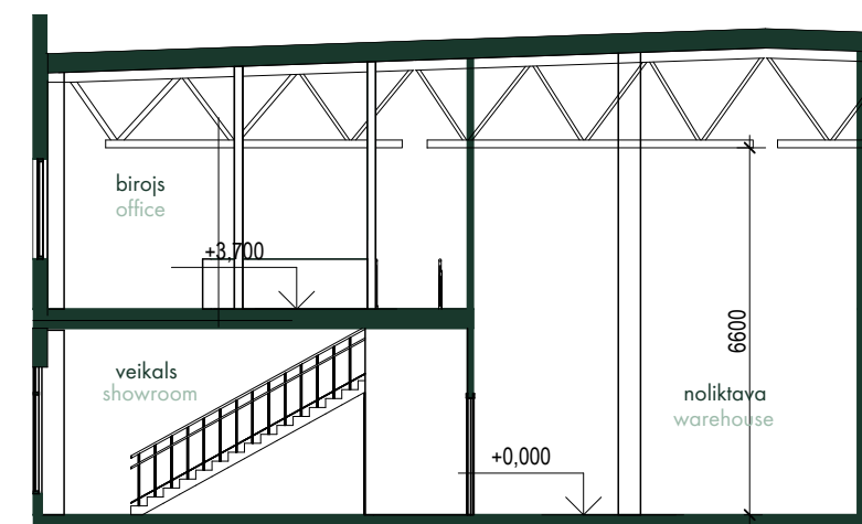
ŠĶĒRSGRIEZUMS 1-1 SECTION 1-1
