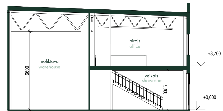
ŠĶĒRSGRIEZUMS 1-1 SECTION 1-1
