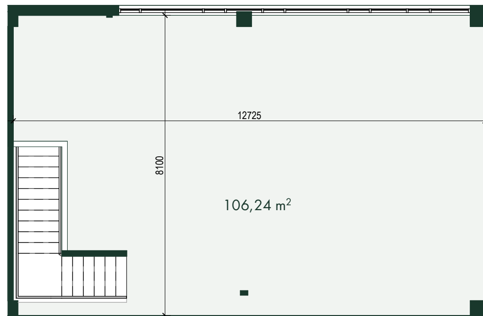
2. STĀVA PLĀNS 2. FLOOR PLAN
