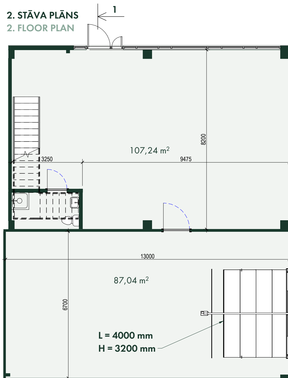
1. STĀVA PLĀNS 1. FLOOR PLAN
