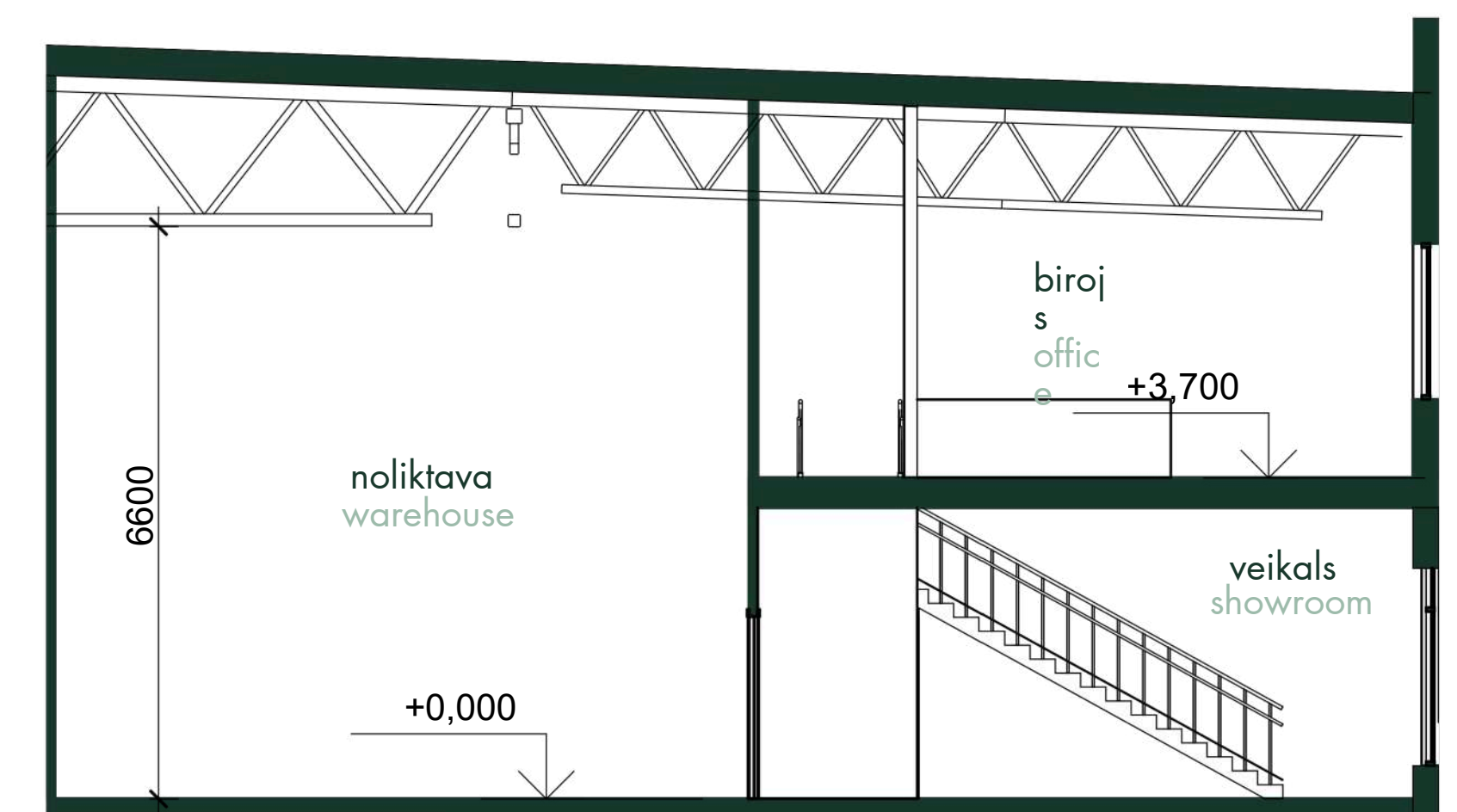
ŠĶĒRSGRIEZUMS 1-1 SECTION 1-1
