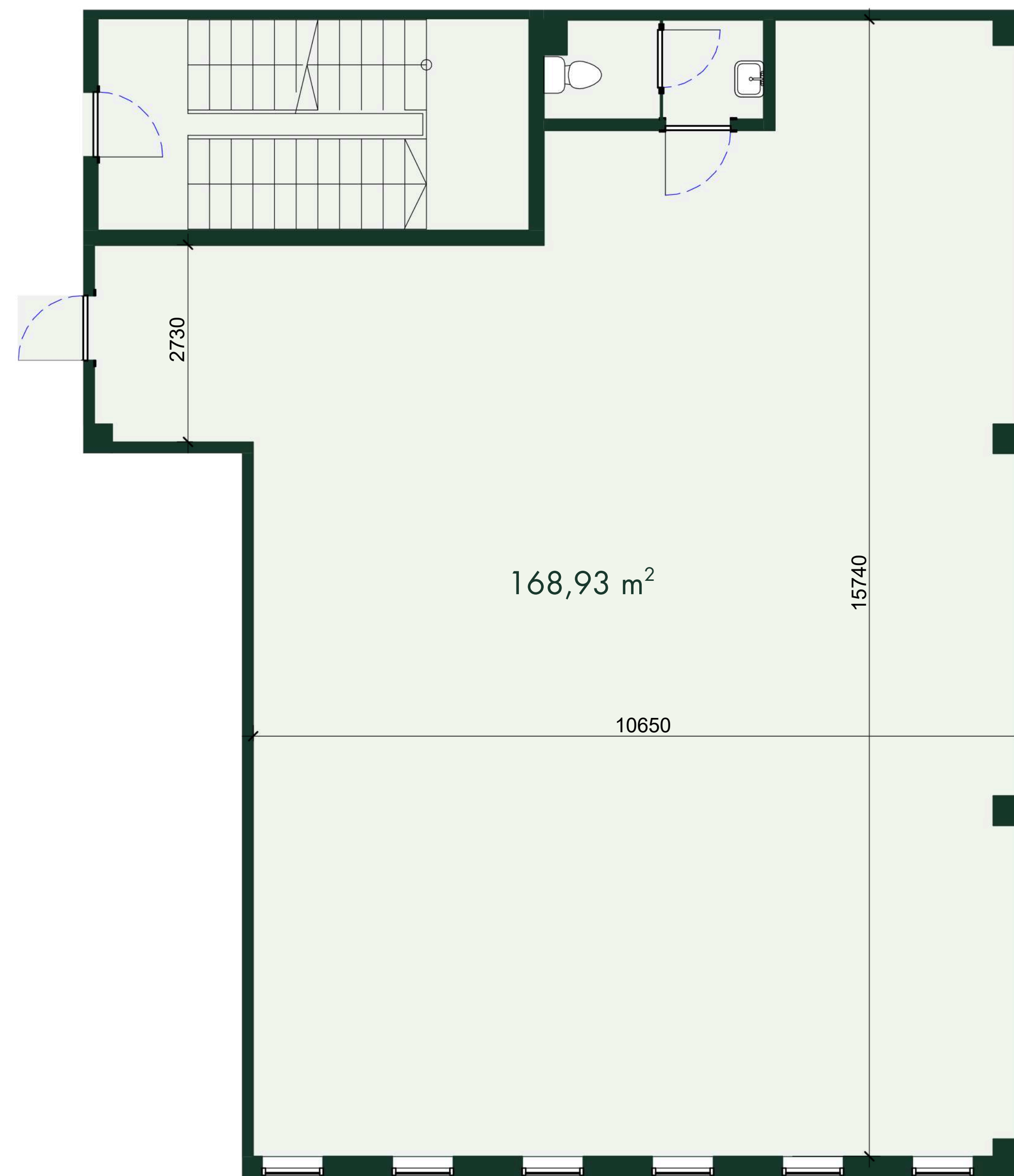
STĀVA PLĀNS FLOOR PLAN
