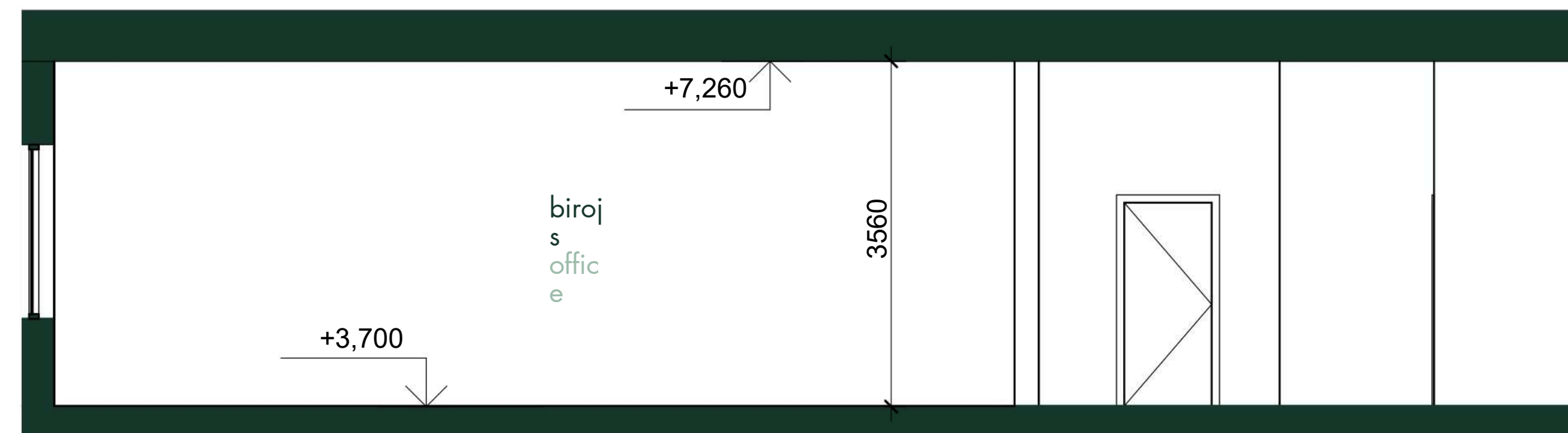
ŠĶĒRSGRIEZUMS 1-1 SECTION 1-1
