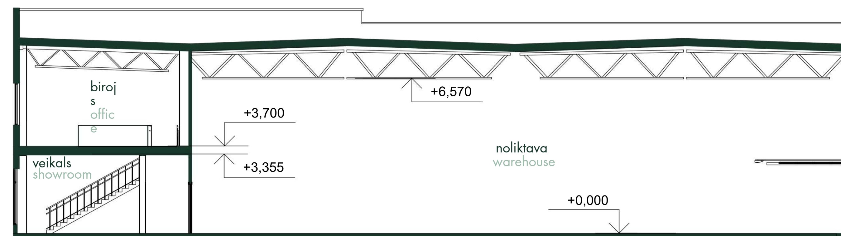
ŠĶĒRSGRIEZUMS 1-1 SECTION 1-1
