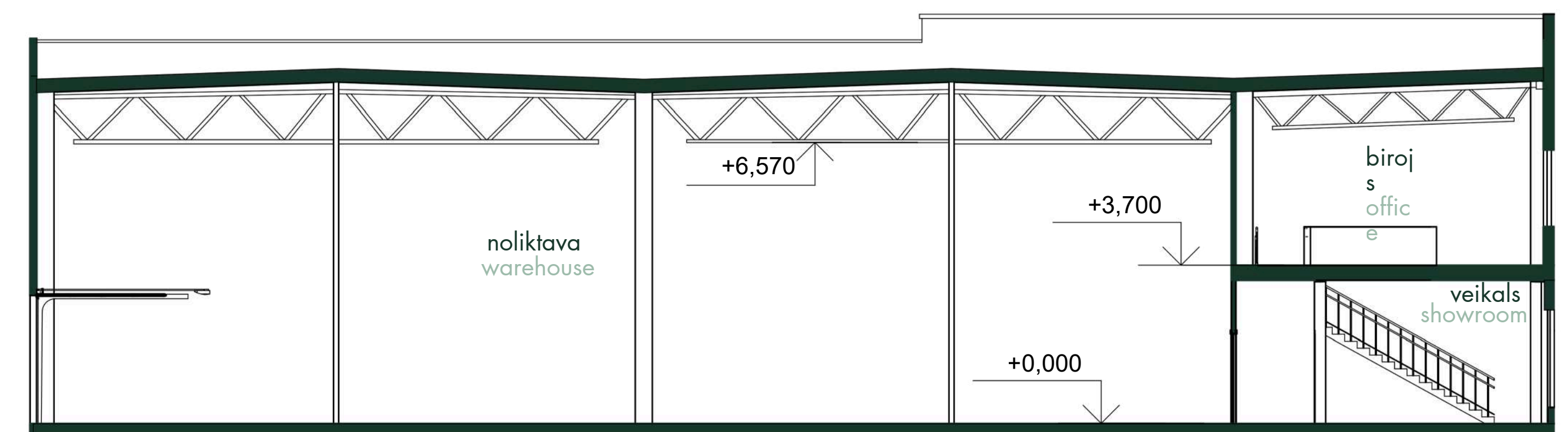
ŠĶĒRSGRIEZUMS 1-1 SECTION 1-1
