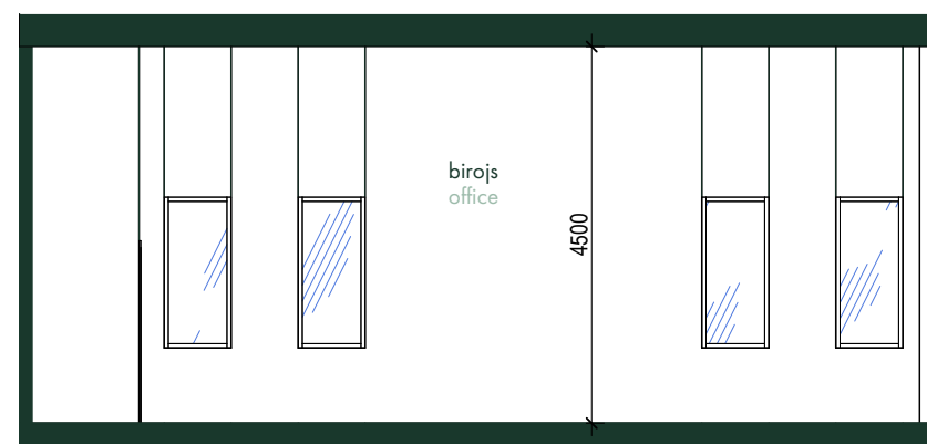
ŠĶĒRSGRIEZUMS 1-1 SECTION 1-1
