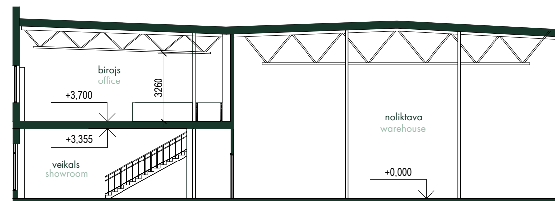
ŠĶĒRSGRIEZUMS 1-1 SECTION 1-1
