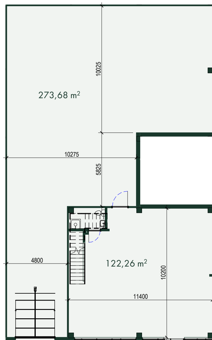
1. STĀVA PLĀNS 1. FLOOR PLAN
