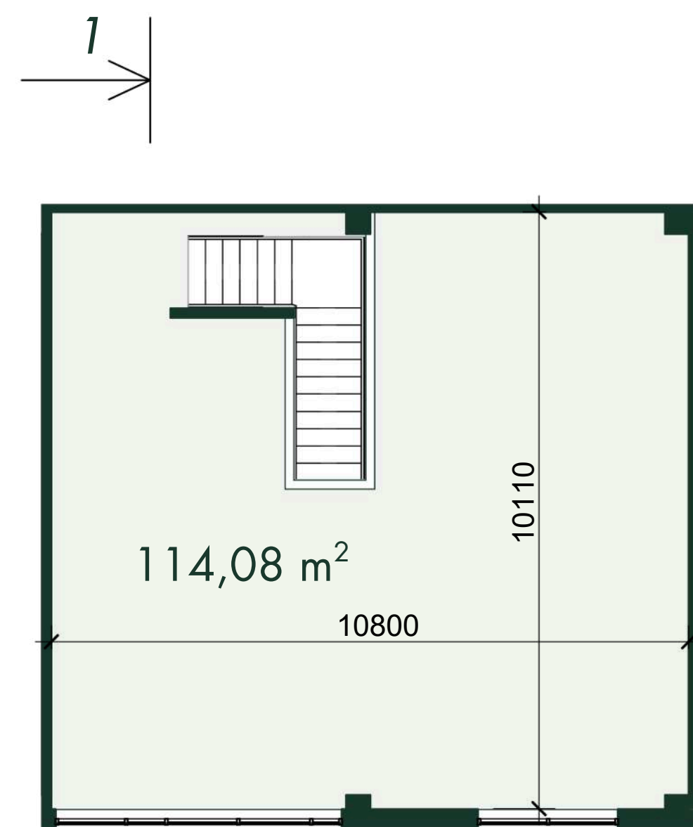
2. STĀVA PLĀNS 2. FLOOR PLAN
