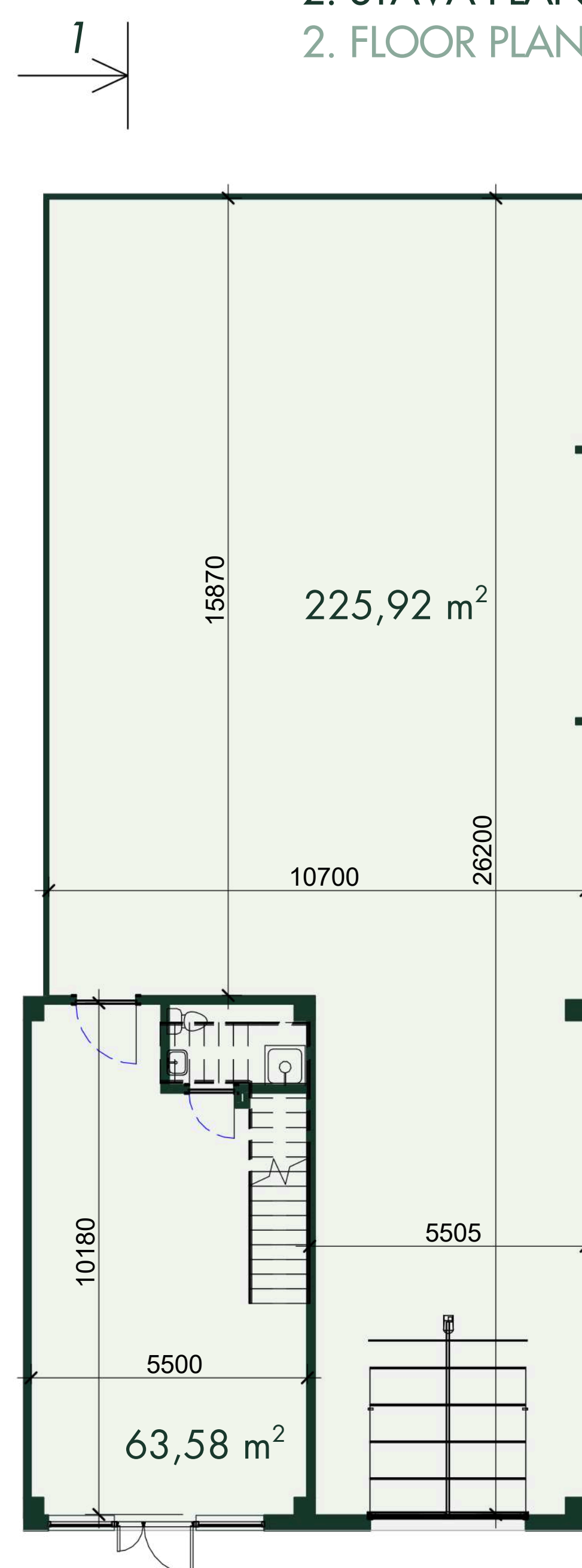
1. STĀVA PLĀNS 1. FLOOR PLAN
