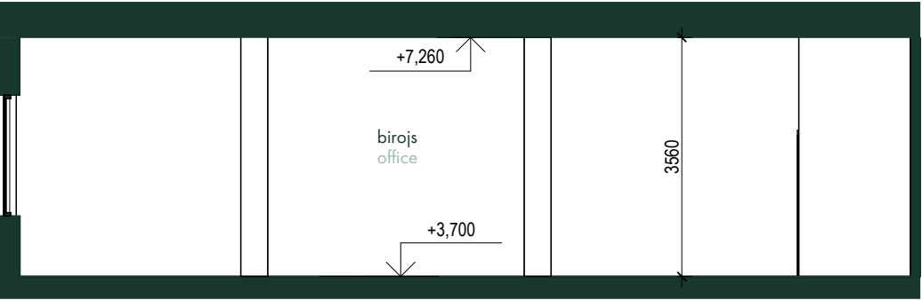
ŠĶĒRSGRIEZUMS 1-1 SECTION 1-1
