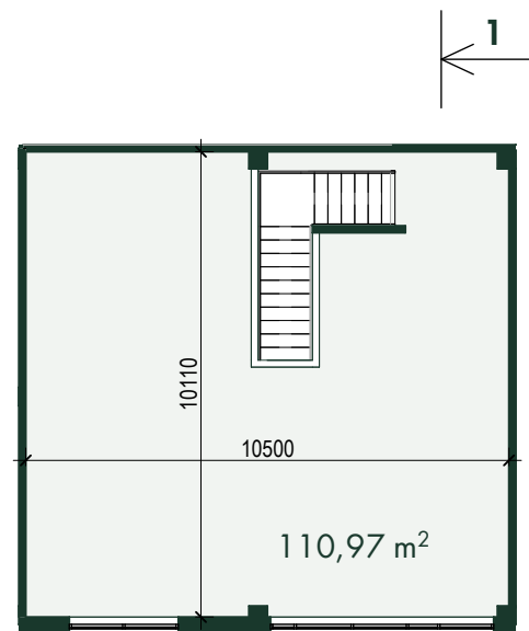
2. STĀVA PLĀNS 2. FLOOR PLAN
